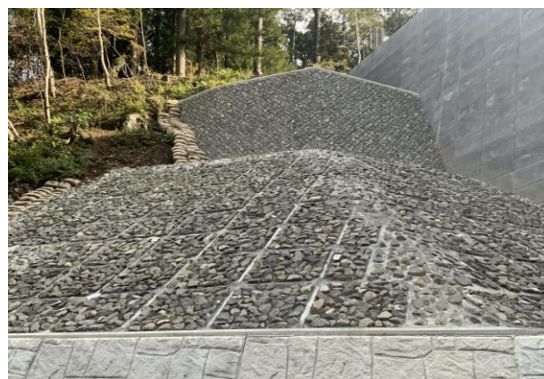
山梨県 富士山宮川砂防
