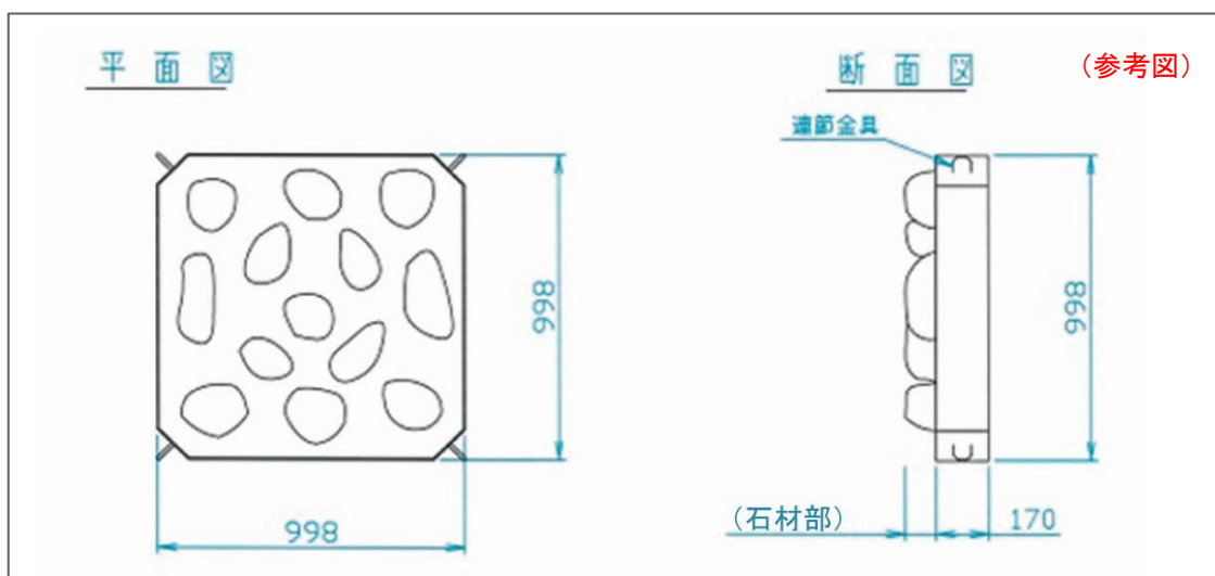
大型連節・張りブロック 玉石 998×998タイプ 350kg以上
